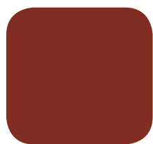
Rouge oxyde
